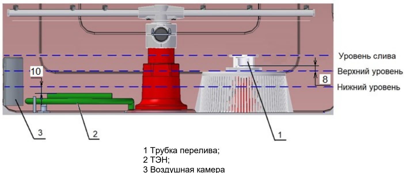
Рис. 4. Уровни воды в ванне
