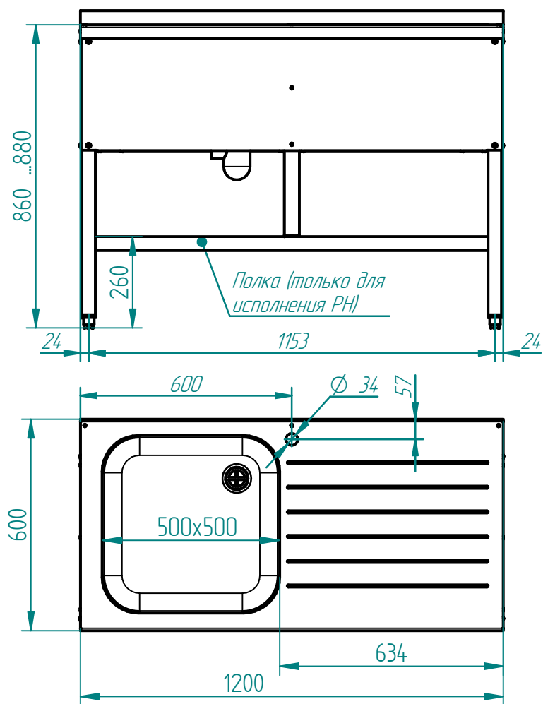
СМО-6-3 РН и СМО-6-3 РЧ
