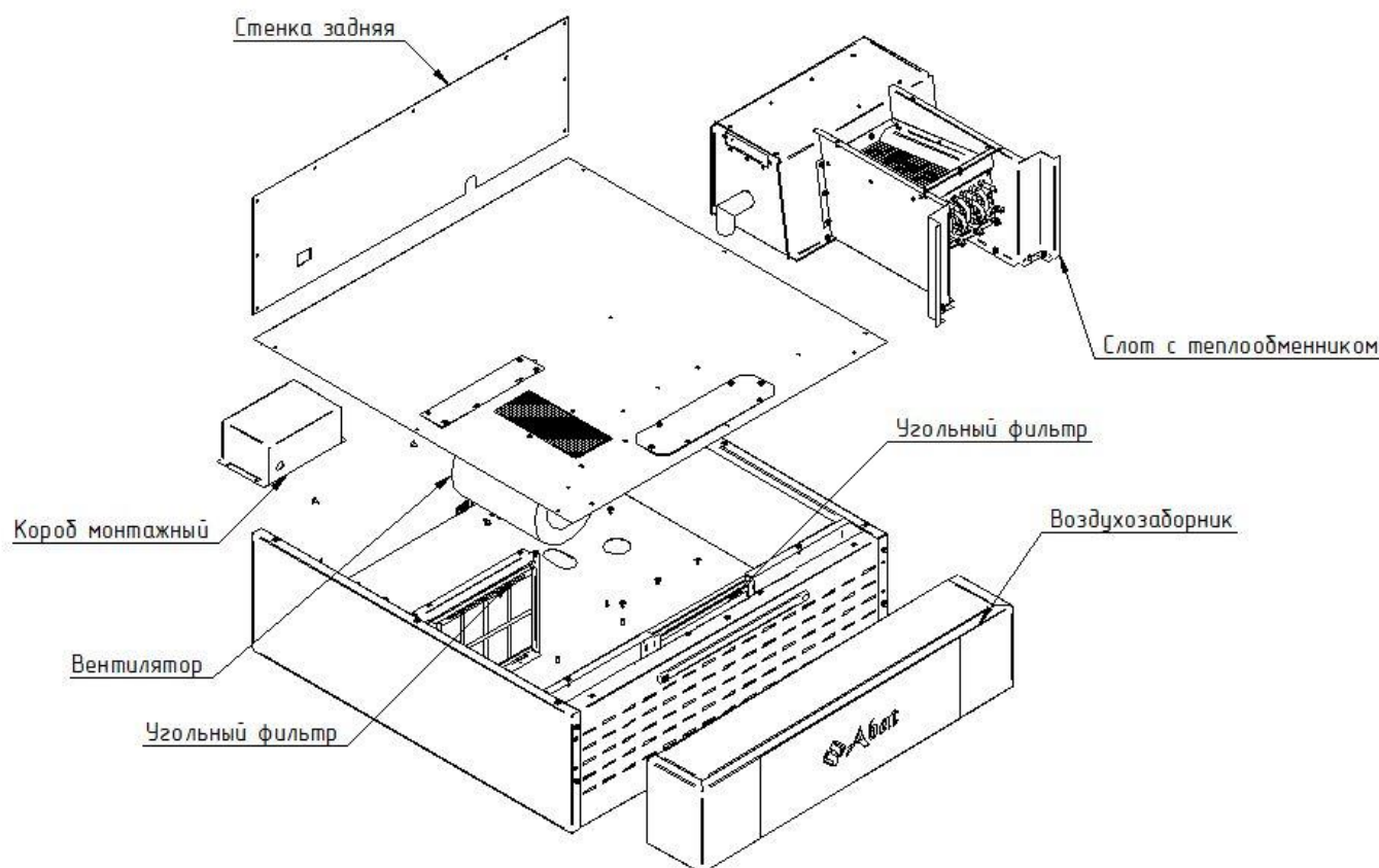
Рис 3 - Состав зонта
