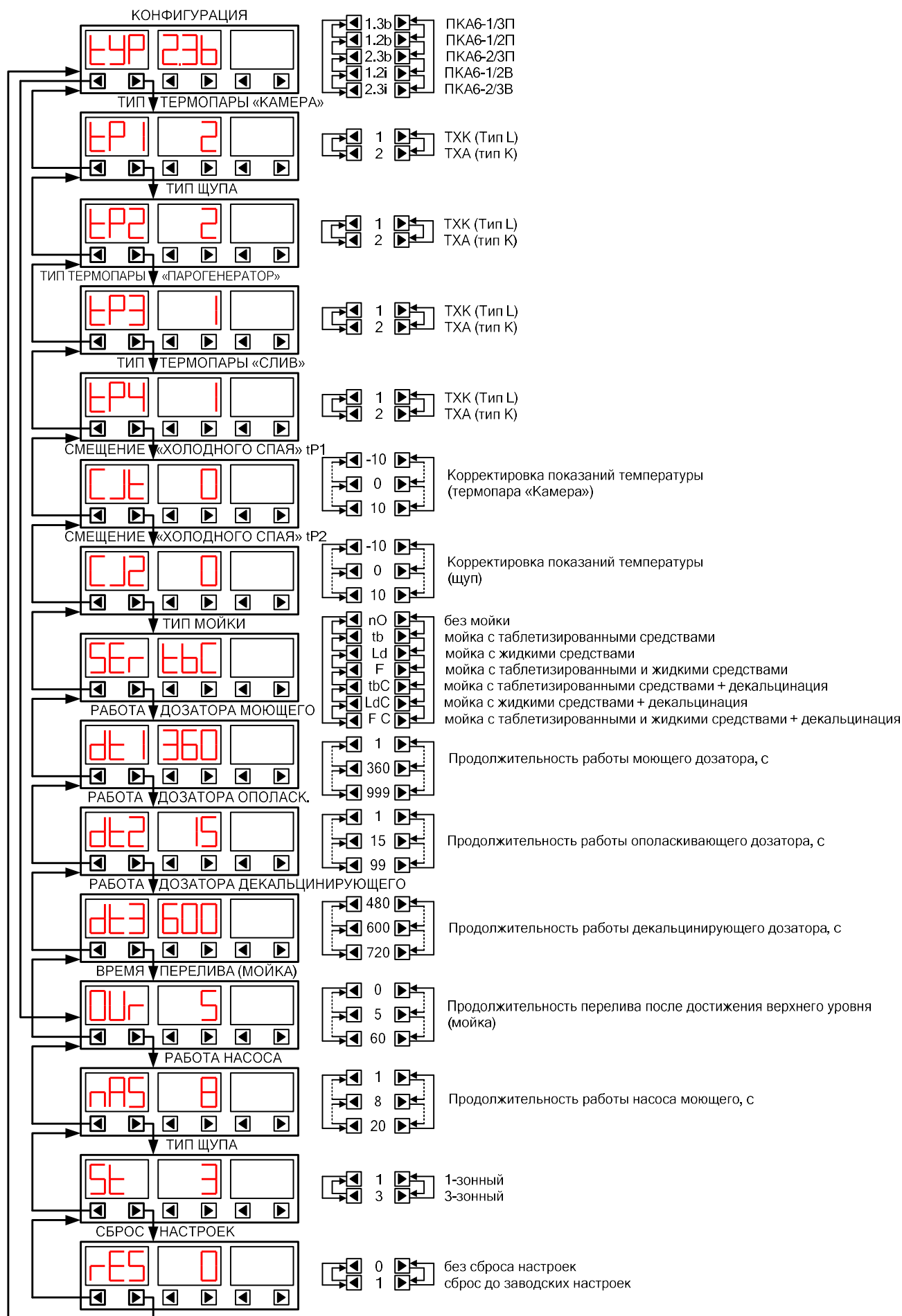
Рис.9. Настройка контроллера
