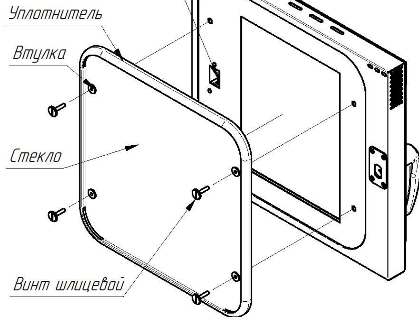
Рис.8. Замена лампы освещения и уплотнителя двери.
